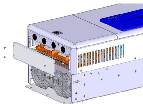
Figura 9: Retirada da chapa de proteção dos cabos nas mecânicas F, G e H
