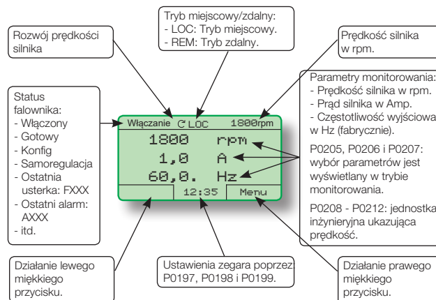
Rysunek 27: Panel z przyciskami i przykłady ustawień fabrycznych (tryb monitorowania)
