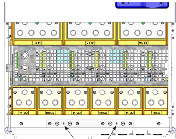
(a) Mecânicas F e G
