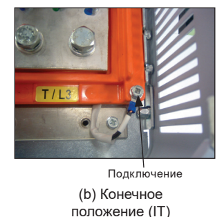
Рис. 21 с (а) до (б): Размеры корпуса F и G с заземлением - расположение и процедура подключения к сети или дельте - переместите фильтр RFI на землю для отключения
