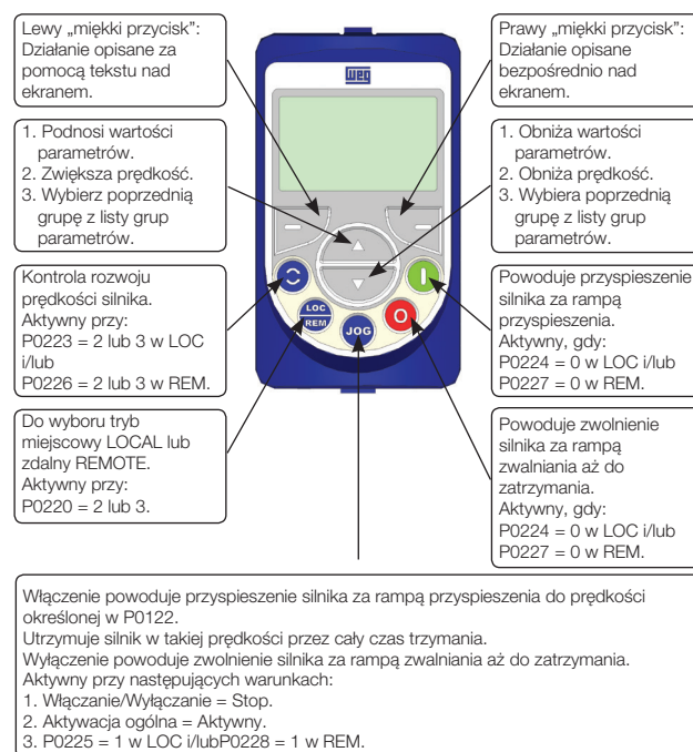
Rysunek 26: Przyciski i ich funkcje
