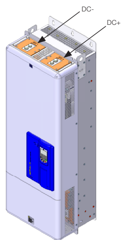
Figura 17 (a) y (b): Terminales de potencia y puesta a tierra de los tamaños F, G y H
