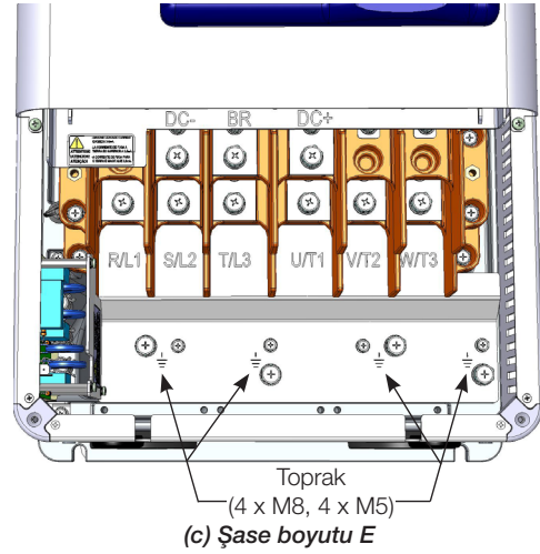
Şekil 16 (a) ila (c): Güç ve topraklama terminaleri şasi boyutu A, B, C, D ve E
