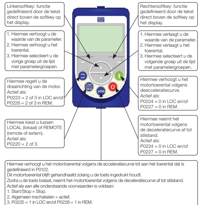
Afbeelding 28: Toetsen van het bedieningspaneel en hun functies
