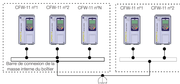
Figure 23: Raccords à la terre de plusieurs variateurs
