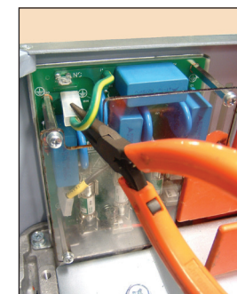
Рис. 20 с (а) до (с): Размеры корпуса Е с заземлением - расположение и порядок подключения к сети или дельте - переместите фильтр RFI на землю для отключения
