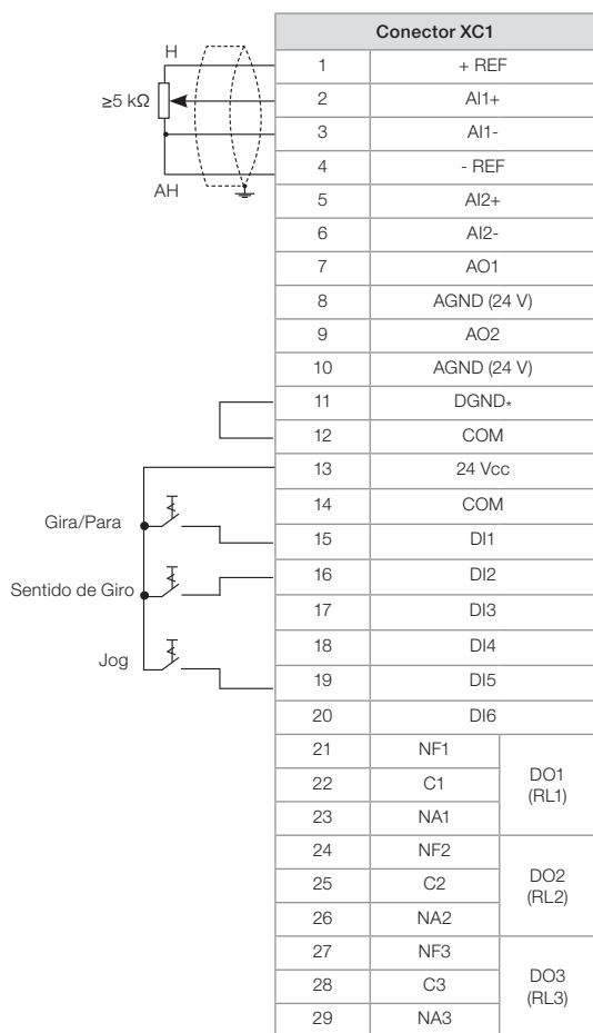
Figura 26: Conexões em XC1 para acionamento 2
