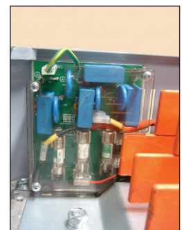
Рис. 20 с (а) до (с): Размеры корпуса Е с заземлением - расположение и порядок подключения к сети или дельте - переместите фильтр RFI на землю для отключения
