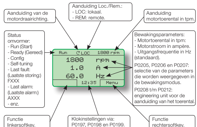
Afbeelding 29: Display van het bedieningspaneel en voorbeeld van standaardfuncties af fabriek (bewakingsmodus)
