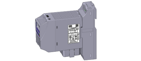
(c) Fit the lower snaps of the filter set into the CFW100 base (c) Encaje las trabas inferiores del conjunto filtro en la base del CFW100 (c) Encaixe as travas inferiores do conjunto filtro na base do CFW100
