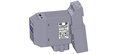
(b) Fit the upper snaps of the filter set into the CFW100 base (b) Encaje las trabas superiores del conjunto filtro en la base del CFW100 (b) Encaixe as travas superiores do conjunto filtro na base do CFW100
