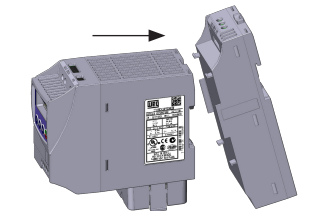
(a) Position the filter set on the CFW100 base (a) Posicione el conjunto filtro en la base del CFW100 (a) Posicione o conjunto filtro na base do CFW100
