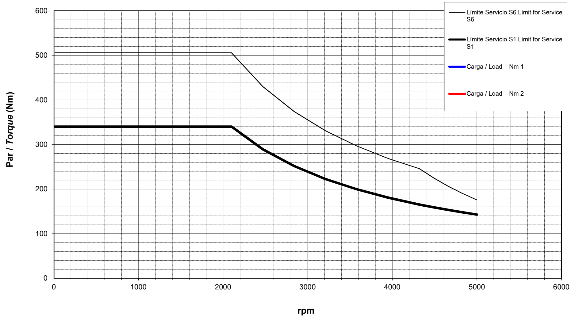
Curva de Par / Torque Diagram
