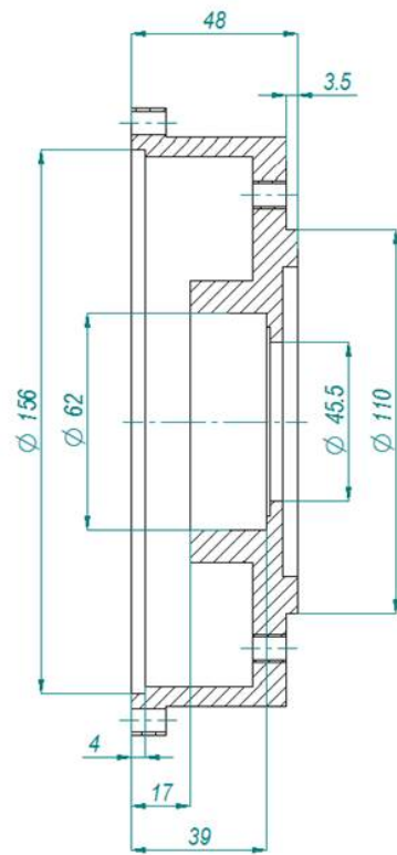
CORTE A-A
