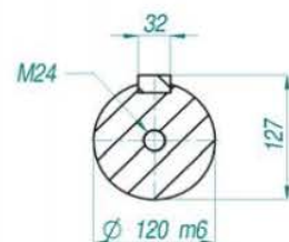
CORTE A-A
