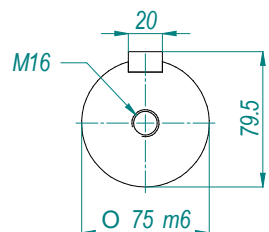
CORTE A-A
