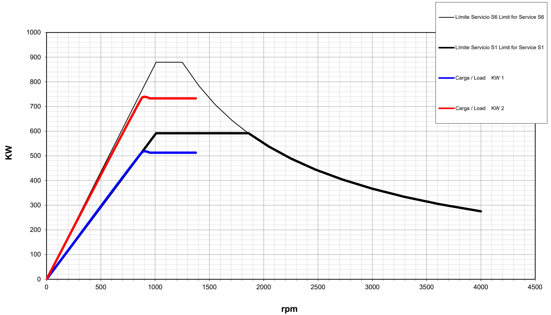
Curva de Potencia / Power Diagram
