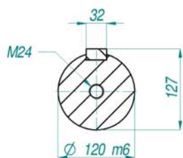
CORTE A-A
