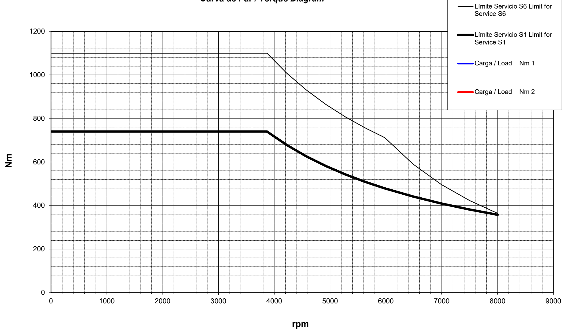
Curva de Par / Torque Diagram
