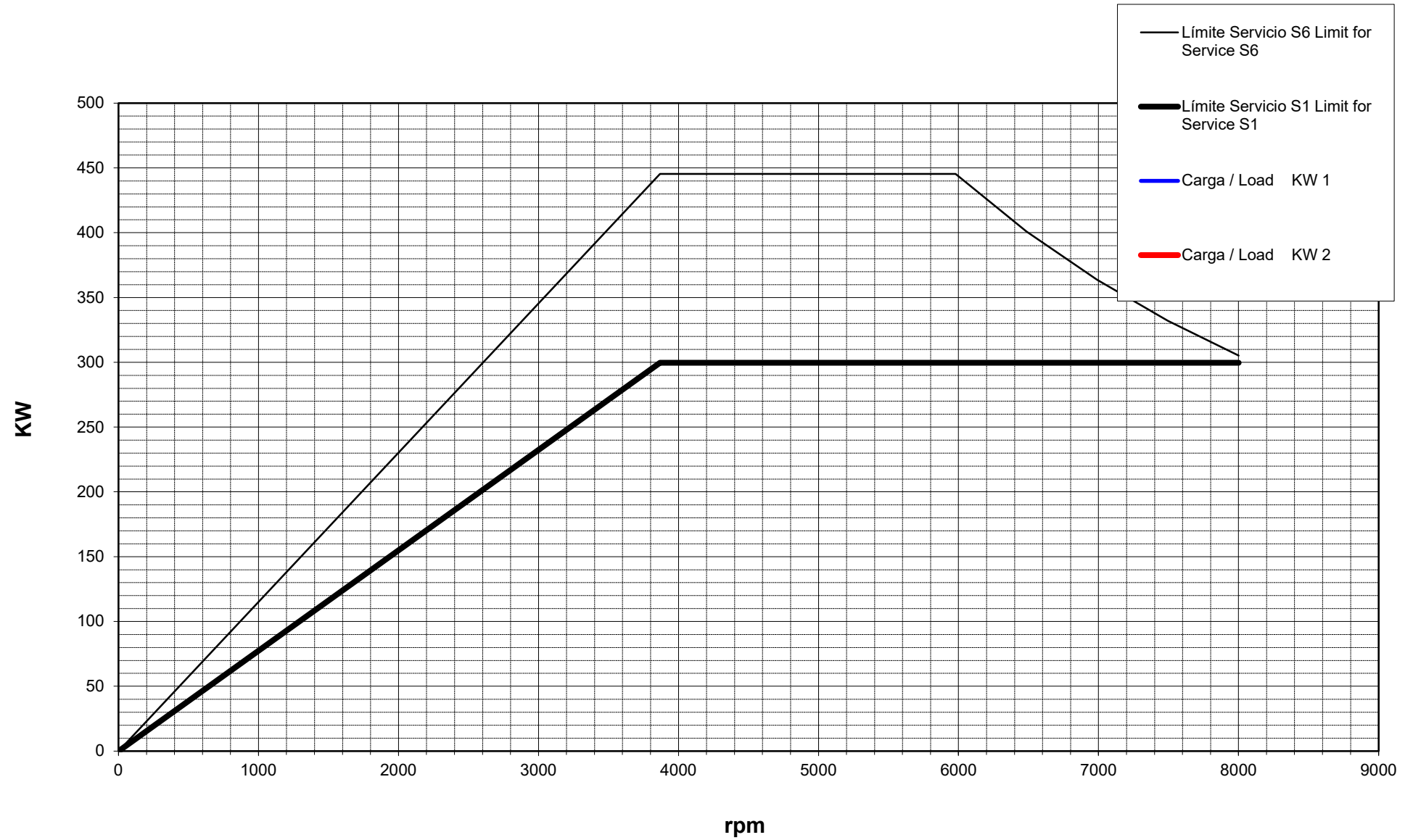
Curva de Potencia / Power Diagram
