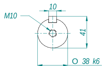
CORTE A-A
