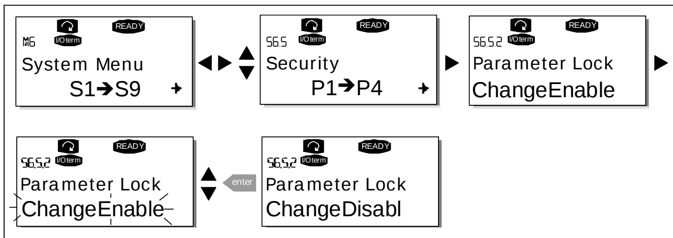
Figure 7-11. Parameter locking
