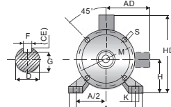
Frame Size 63-200
