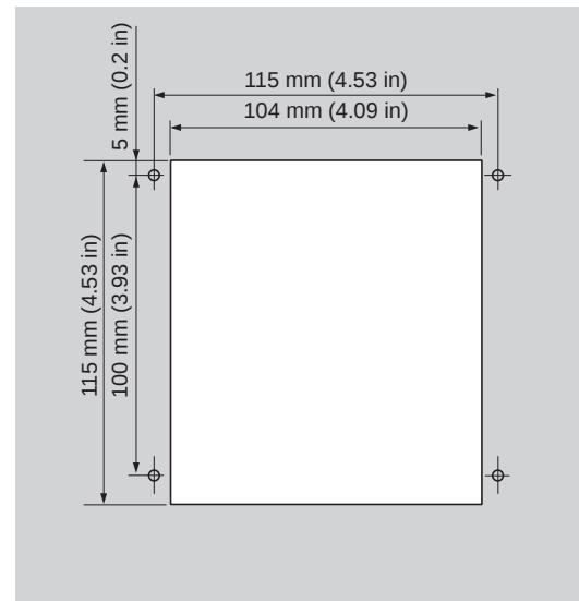
ATV 61
