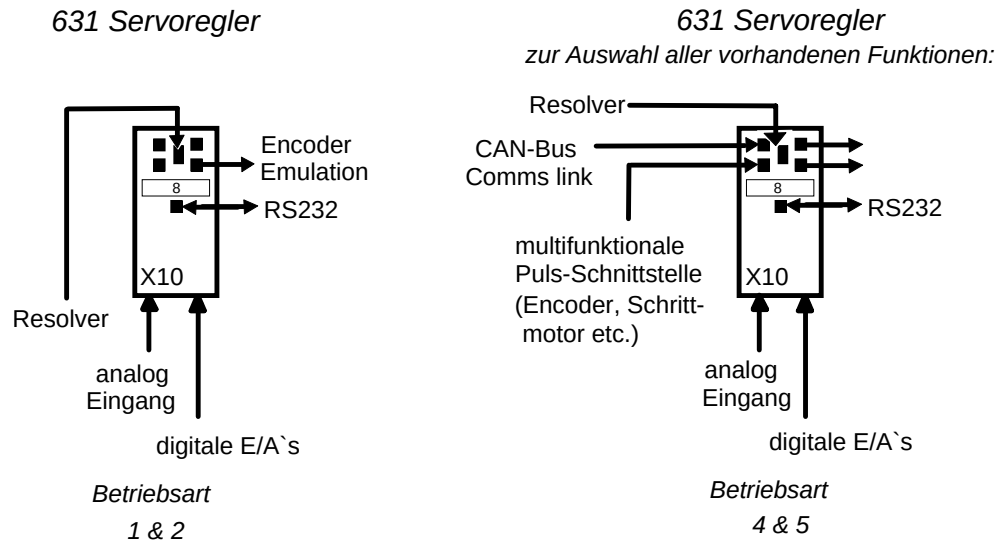
Abbildung 4-1 Anschlussbeispiele
