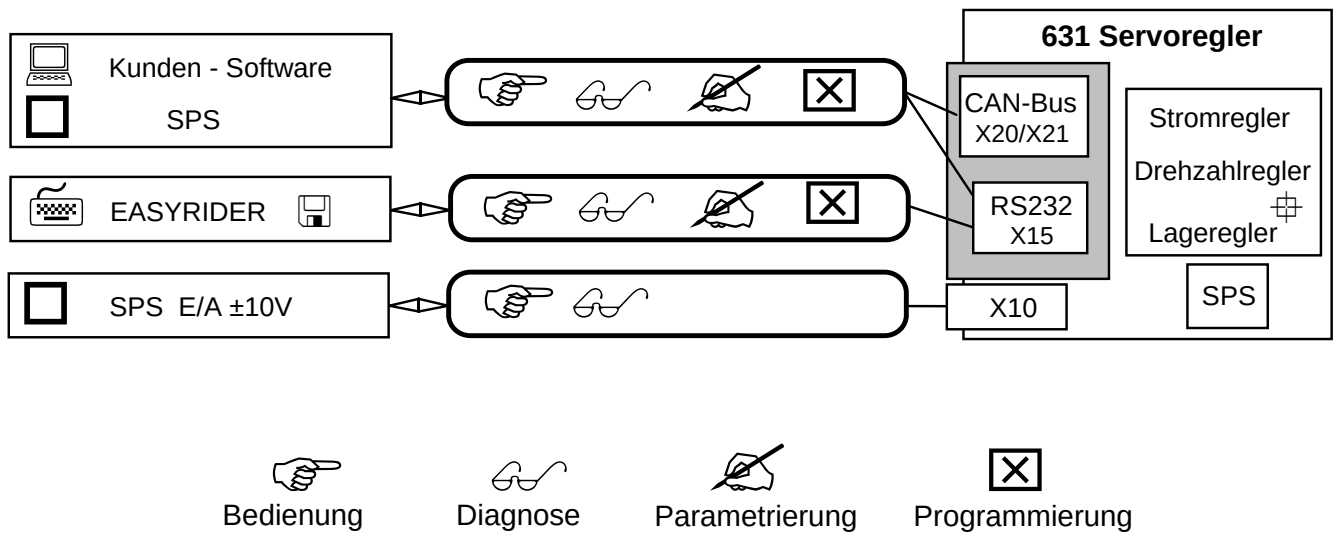
Abbildung 2-2 Digitale Kommunikation
