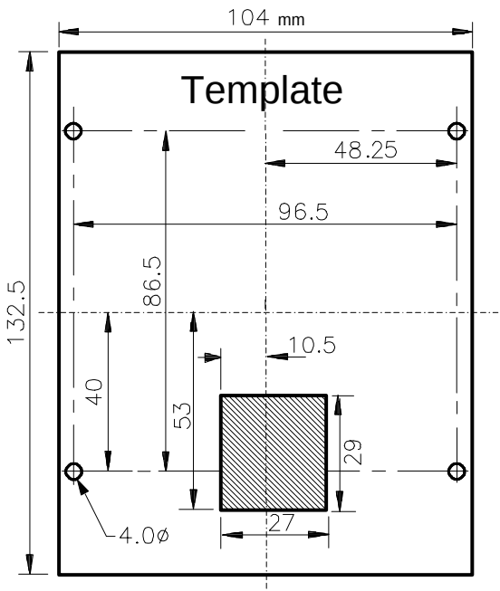
Frequenzumrichter 650 Baugröße 1, 2 & 3
