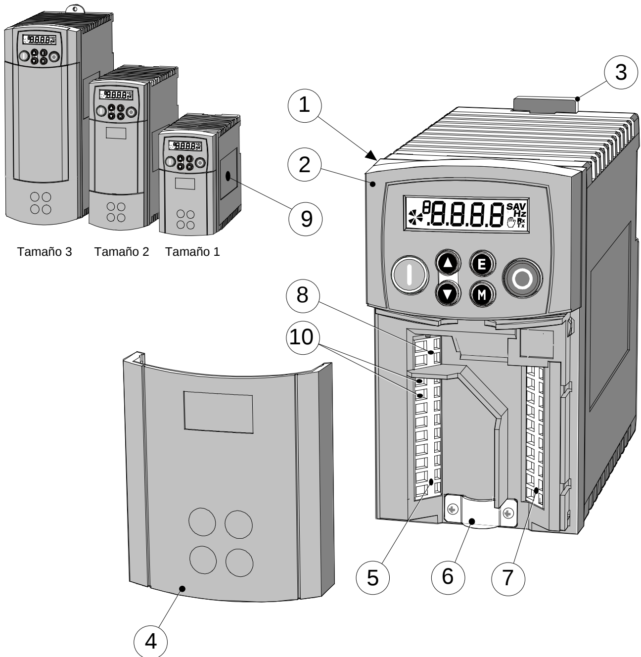
Figure 2-Error! Unknown switch argument. Vista de Partes de Componentes (Tamaño 1 Ilustrado)
