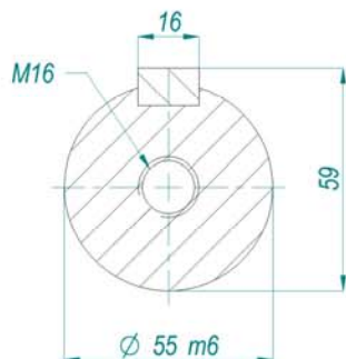
CORTE A-A
