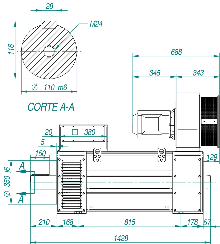
MAC -QE/QI 250 X Motor Dimensions
