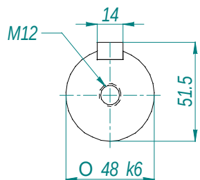
CORTE A-A
