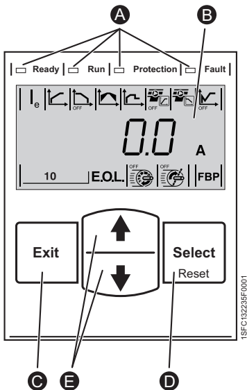
Kuva 5.1: Käyttöliittymä (HMI)
